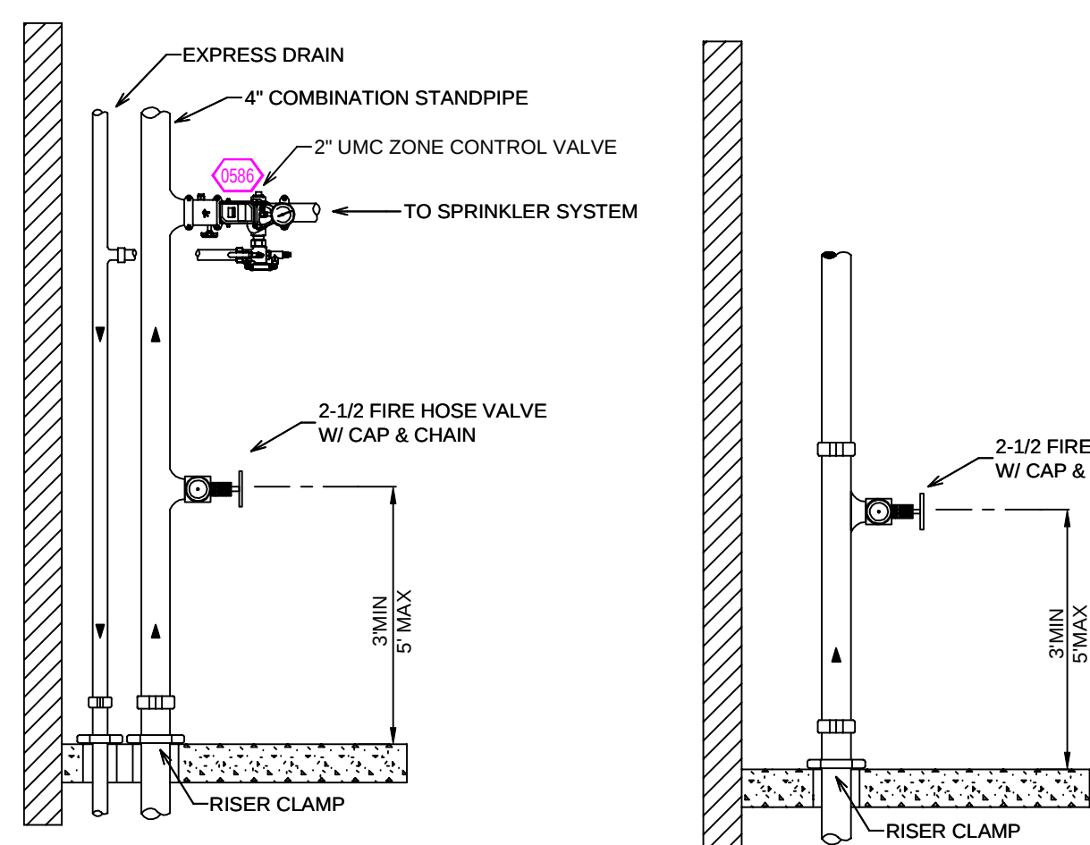
STAIR 2 SP SECTION SCALE: 1/2" = 1'-0" STAIR 1 SP SECTION SCALE: 1/2" = 1'-0"
